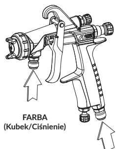
POWIETRZE (Kubek/Ciśnienie)
